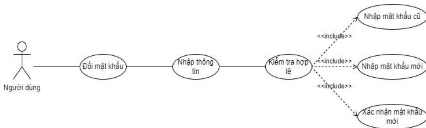
Hình 21. UseCase đổi mật khẩu
