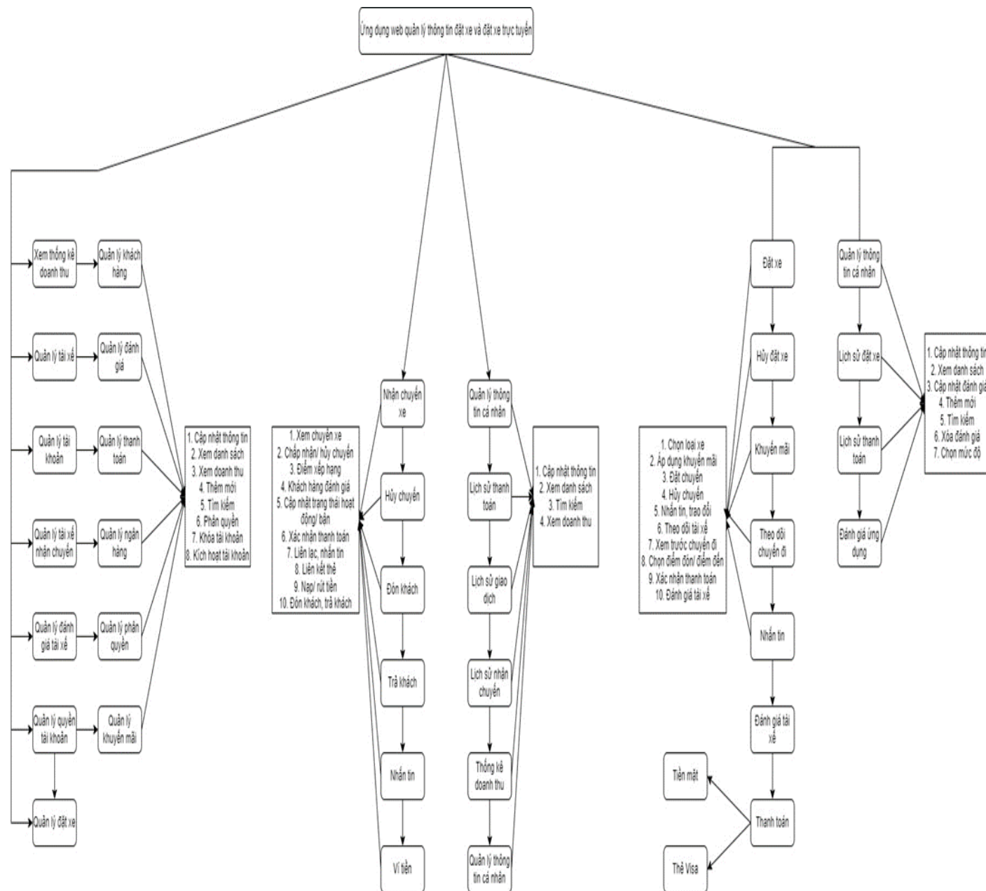
Hình 61. Sơ đồ BFD
