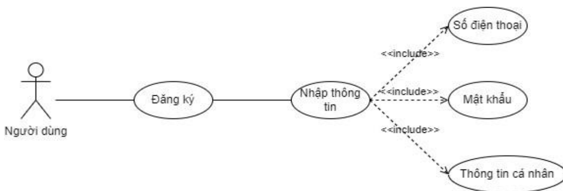
Hình 19. UseCase Đăng ký
