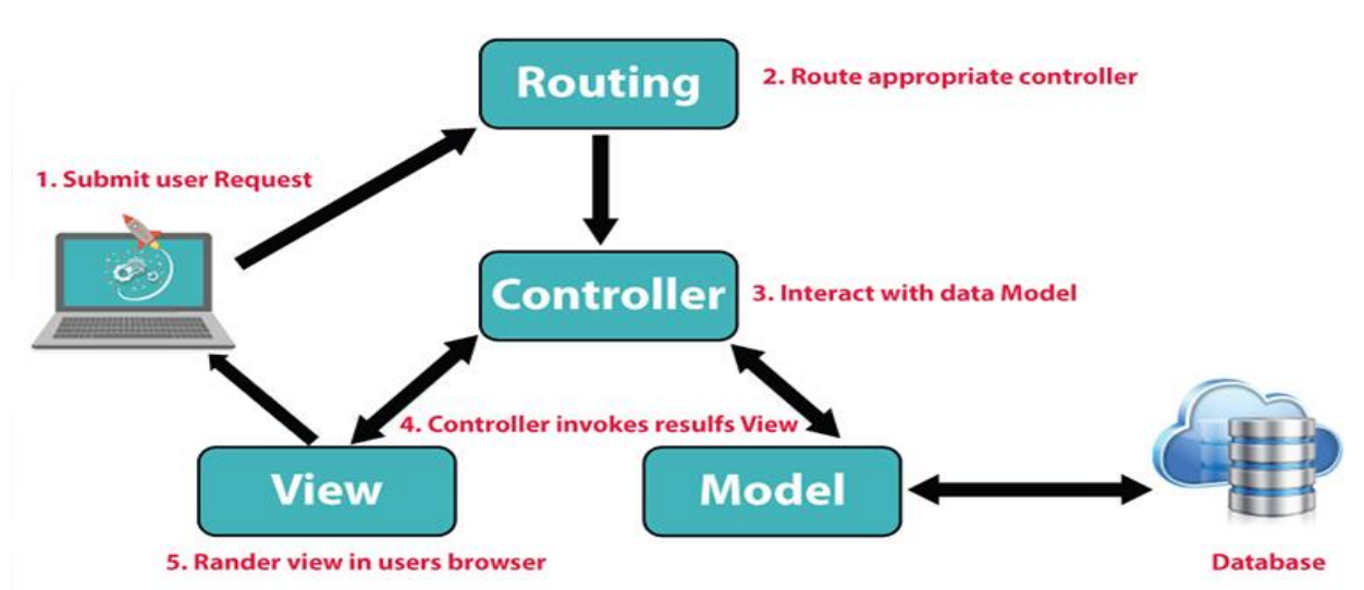
Hình 6. Mô hình MVC
