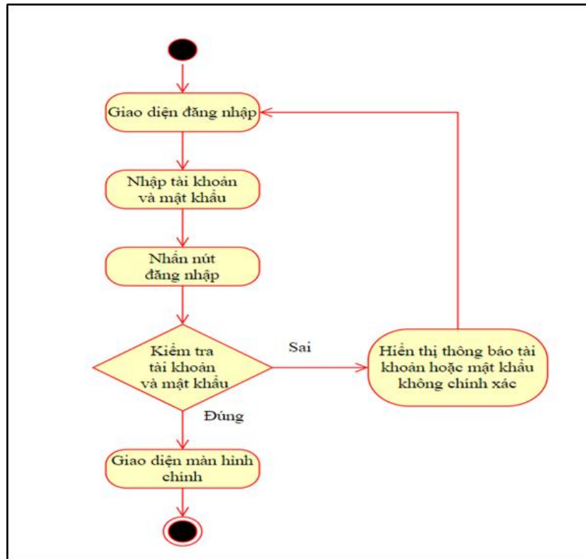
Hình 48. Sơ đồ bản vẽ hoạt động đăng nhập
