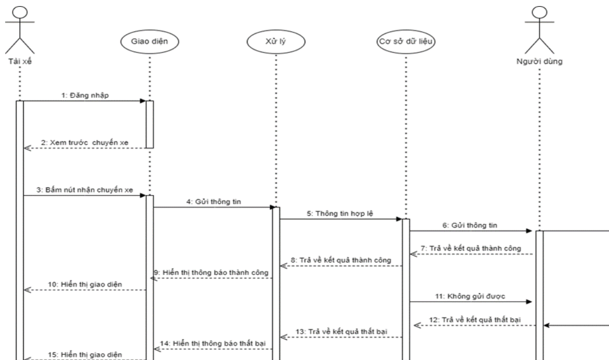
Hình 41. Sơ đồ tuần tự tài xế nhận chuyến xe
