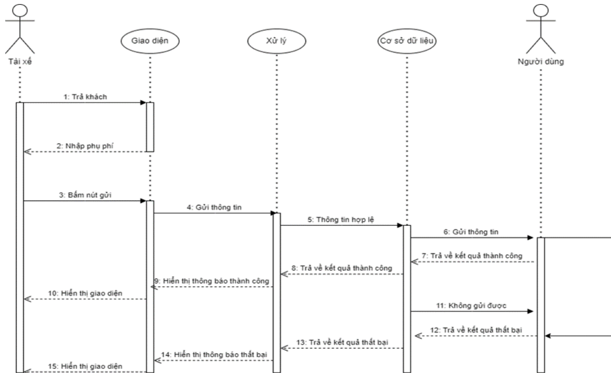
Hình 45. Sơ đồ tuần tự thanh toán và xác nhận hóa đơn
