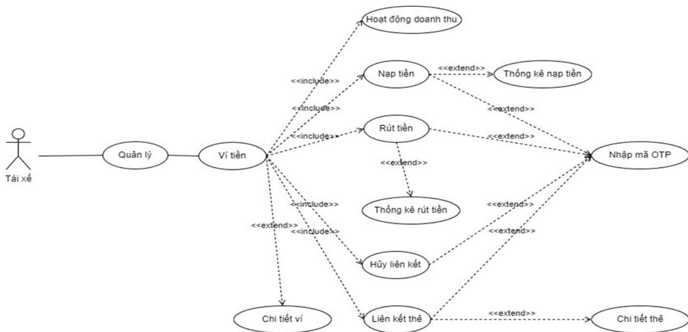
Hình 32. UseCase ví tiền tài xế
