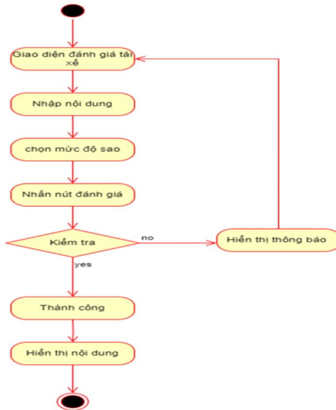
Hình 57. Sơ đồ bản vẽ hoạt động đánh giá tài xế
