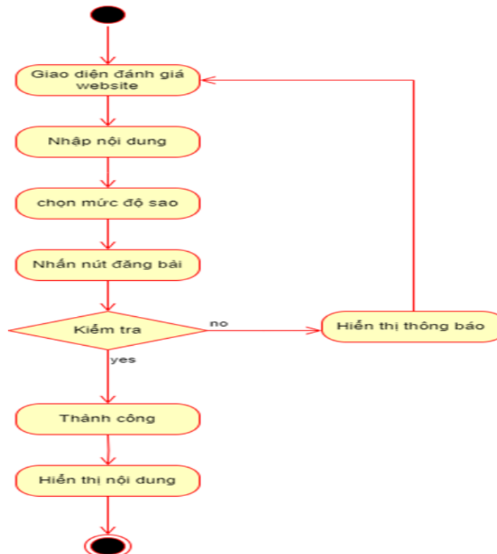
Hình 56. Sơ đồ bản vẽ hoạt động đánh giá ứng dụng web
