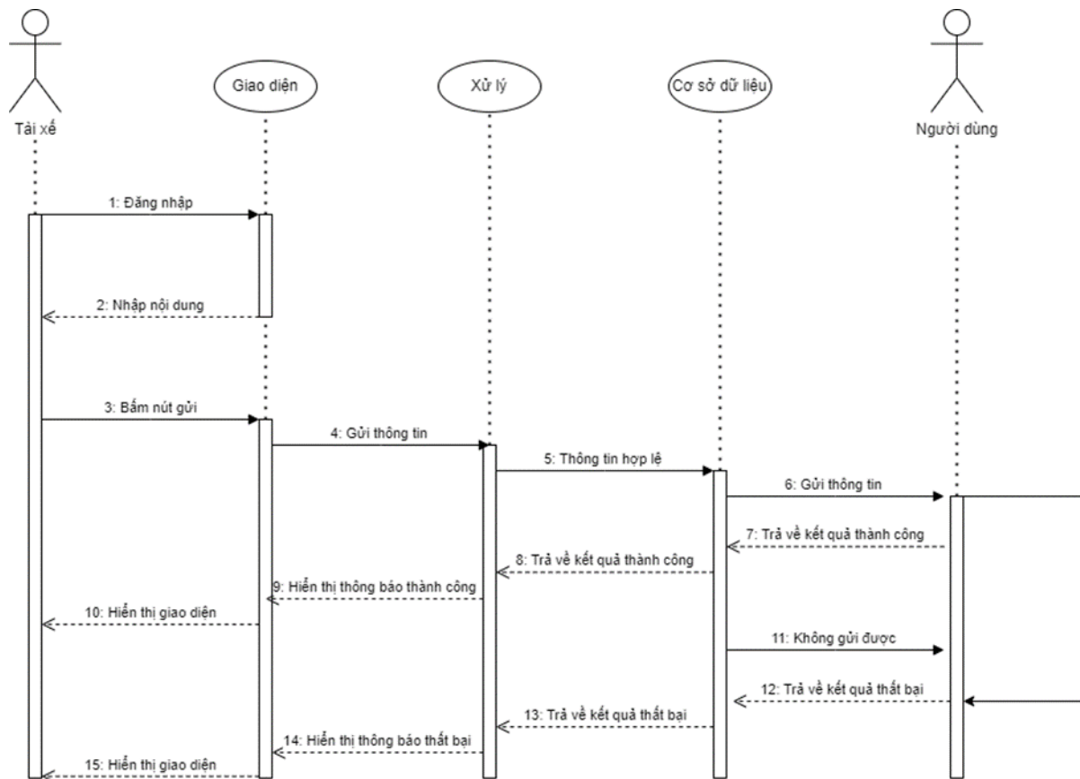
Hình 42. Sơ đồ tuần tự nhắn tin
