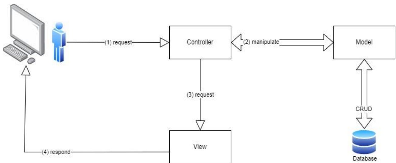
Hình 116. Mô hình MVC của hệ thống
