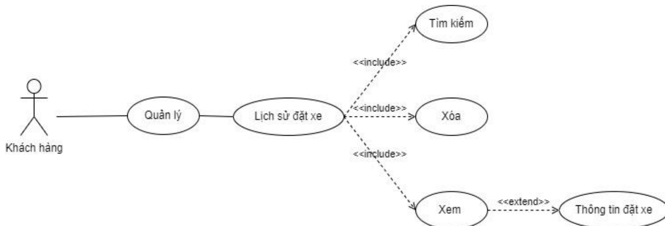
Hình 29. UseCase quản lý lịch sử đặt xe
