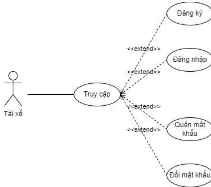
Hình 16. UseCase cấp 0 tài xế
