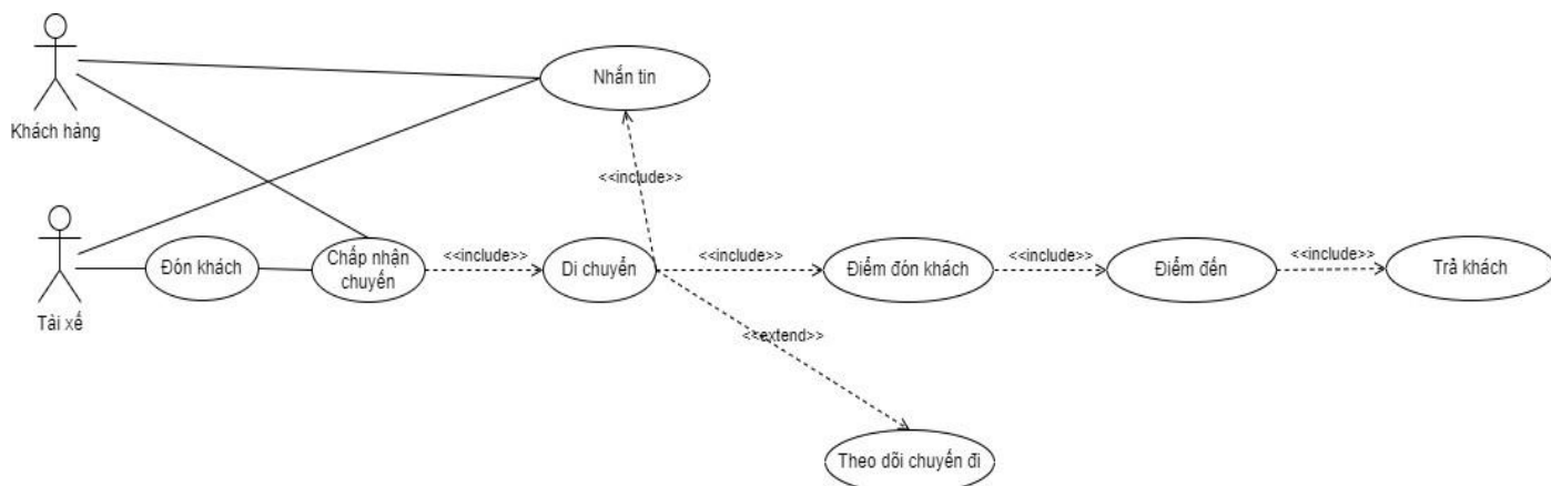
Hình 26. UseCase nhấn tin
