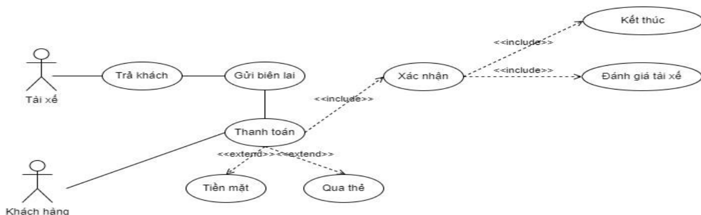
Hình 25. UseCase trả khách
