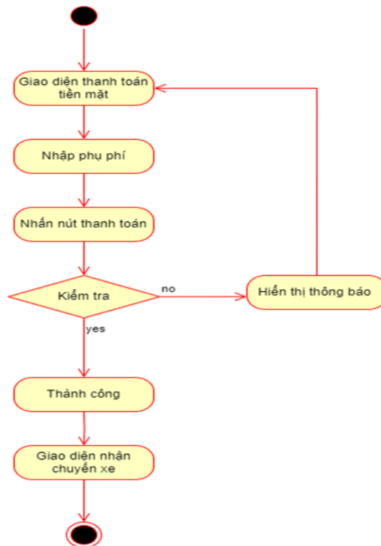
Hình 58. Sơ đồ bản vẽ hoạt động thanh toán và xác nhận hóa đơn
