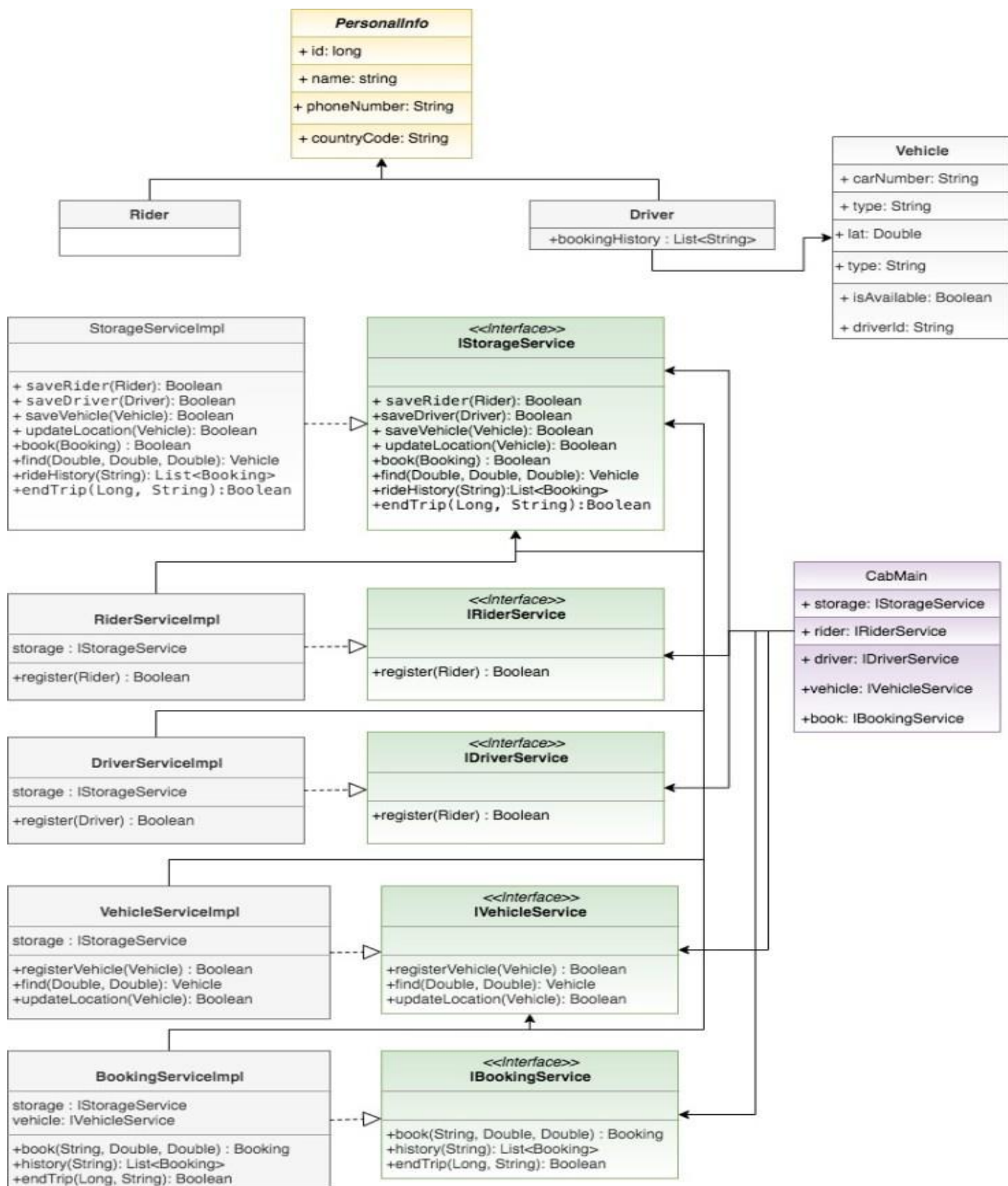
Hình 62. Mô hình Class Diagrams
