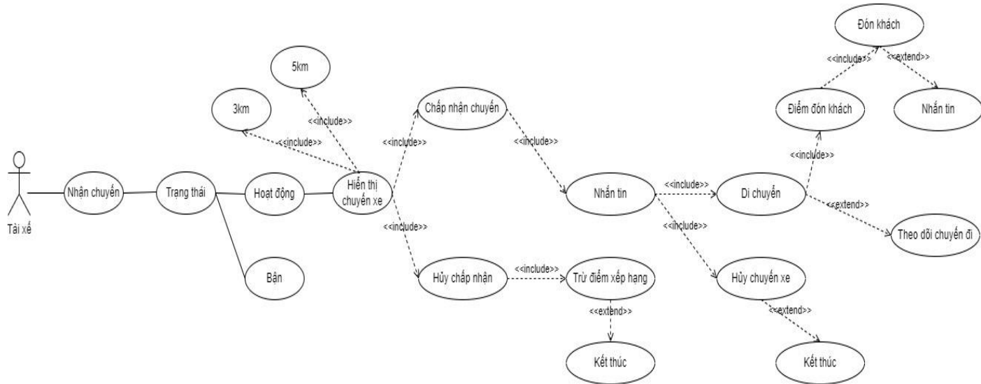
Hình 23. UseCase nhận chuyển xe
