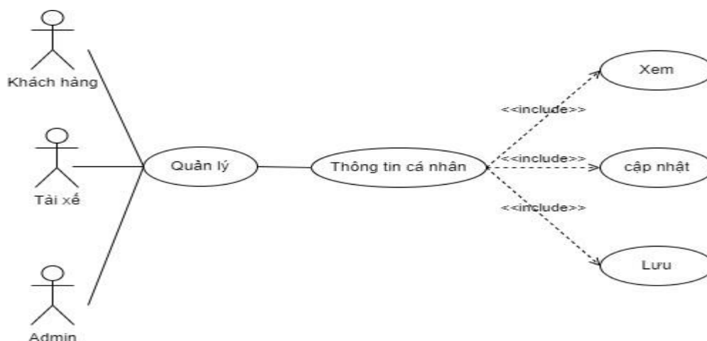
Hình 27. UseCase quản lý thông tin cá nhân
