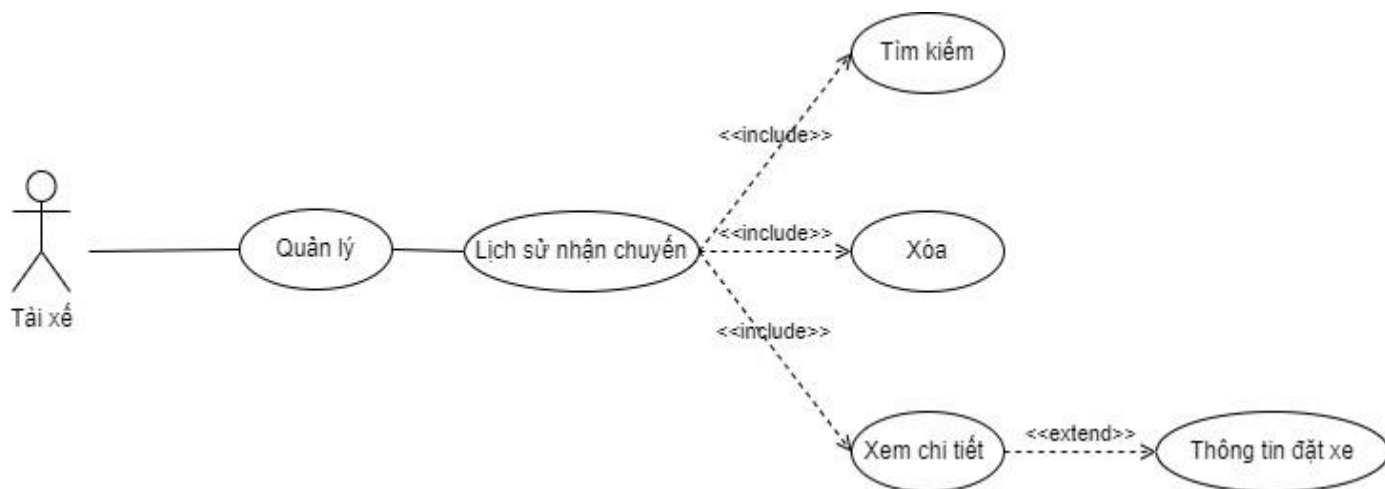
Hình 30. UseCase quản lý lịch sử nhận chuyến xe
