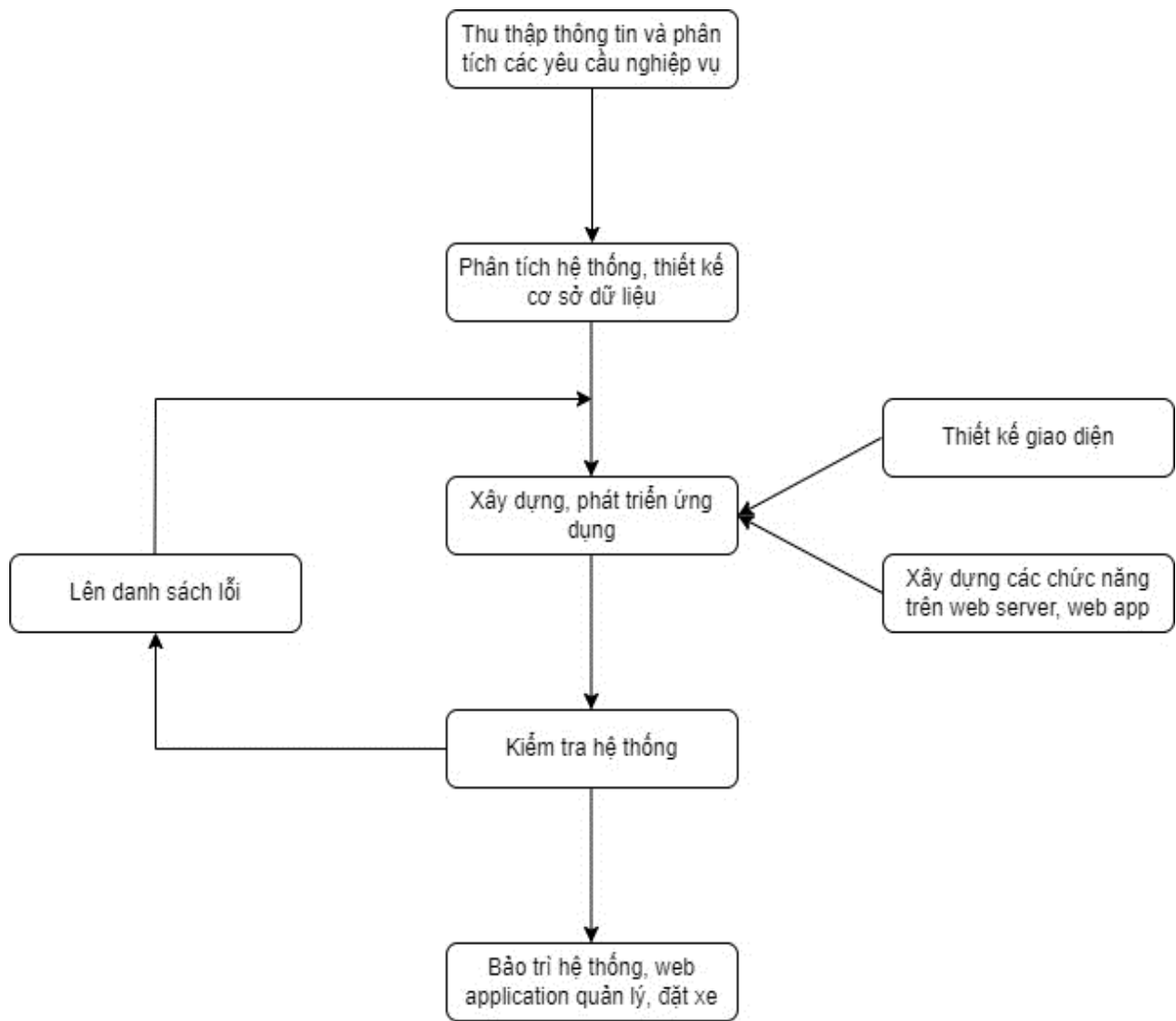
Hình 8. Mô hình phát triển hệ thống
