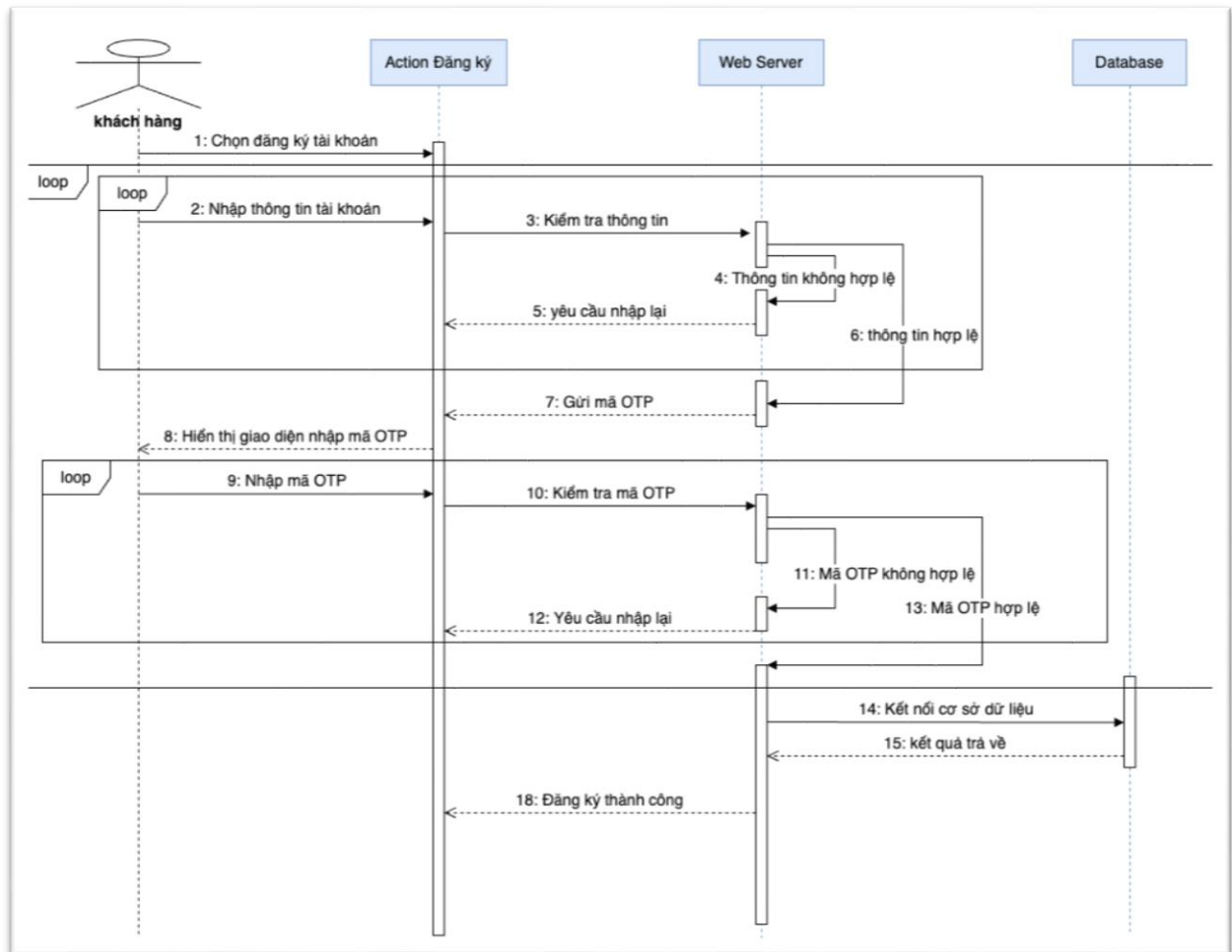
Hình 38. Sơ đồ tuần tự đăng ký
