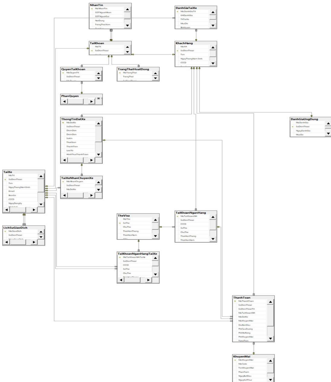
Hình 63. Mô hình cơ sở dữ liệu quan hệ
