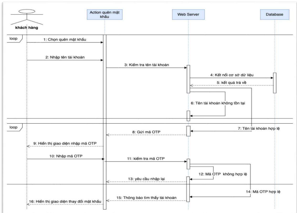
Hình 39. Sơ đồ tuần tự quên mật khẩu
