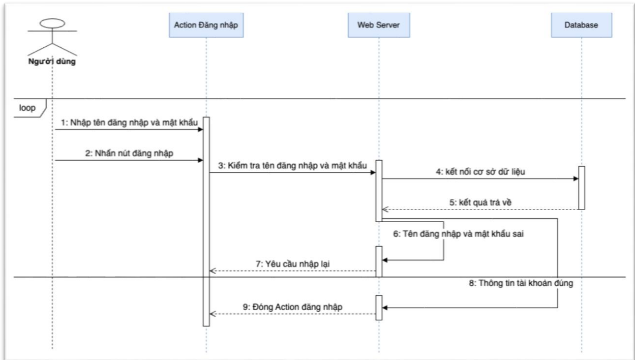
Hình 37. Sơ đồ tuần tự đăng nhập
