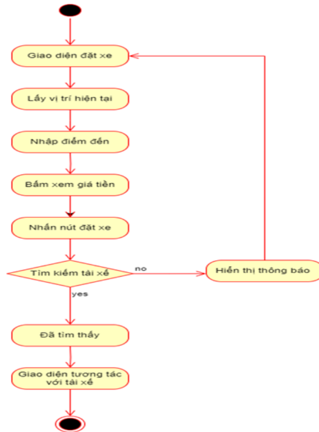
Hình 50. Sơ đồ bản vẽ hoạt động đặt xe
