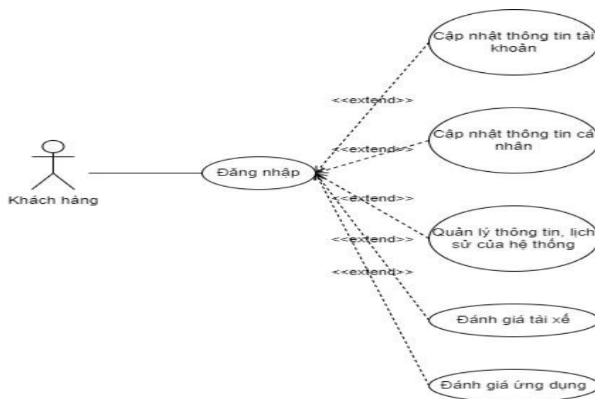
Hình 13. UseCase Cấp 1 khách hàng – Đăng nhập
