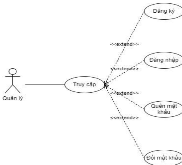
Hình 14. UseCase cấp 0 Quản lý
