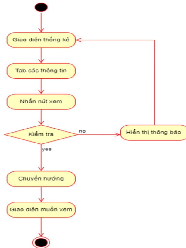
Hình 60. Sơ đồ bản vẽ hoạt động thống kê doanh thu
