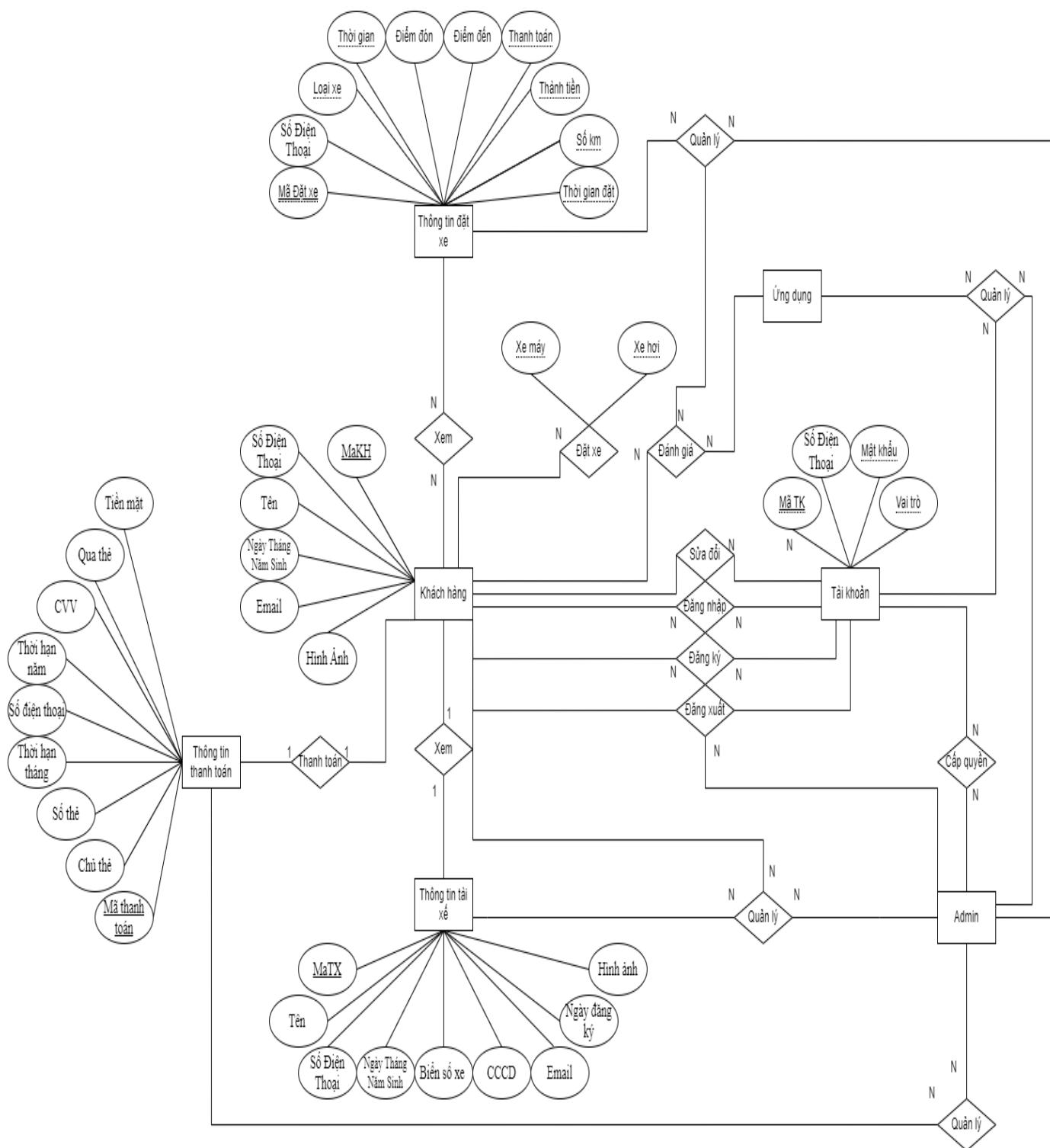
Hình 10. Sơ đồ ERD
