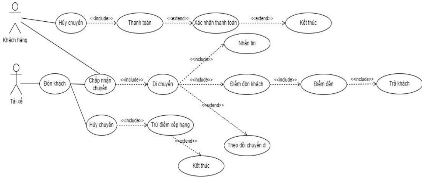
Hình 24. UseCase đón khách
