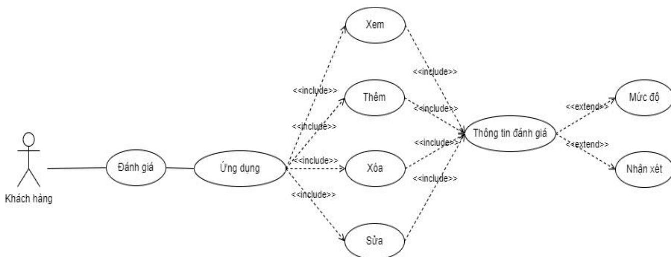
Hình 33. Đặc tả UseCase đánh giá ứng dụng
