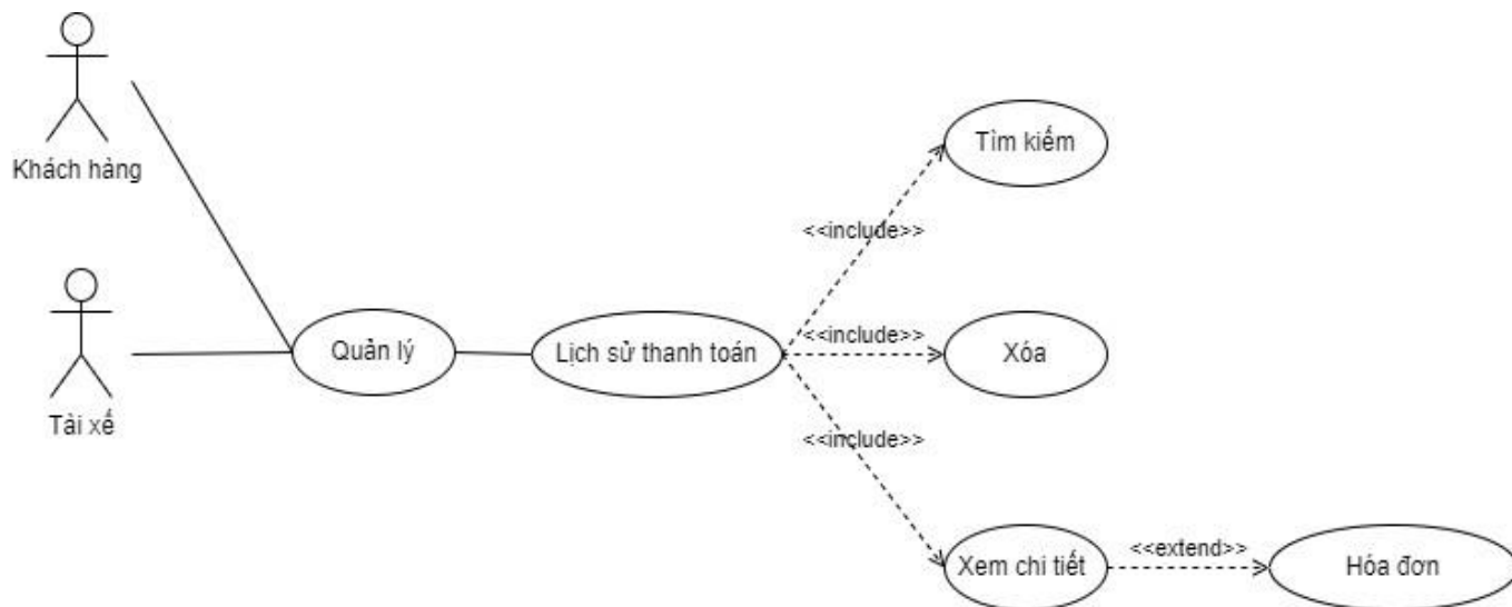
Hình 31. UseCase quản lý lịch sử hóa đơn, thanh toán
