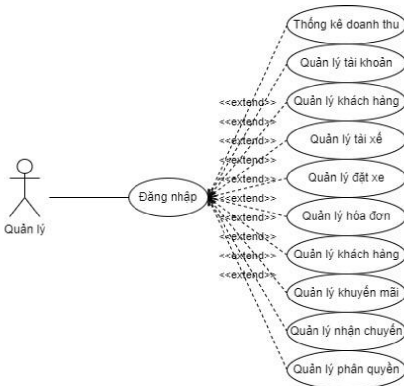
Hình 15. UseCase cấp 1 quản lý – Đăng nhập
