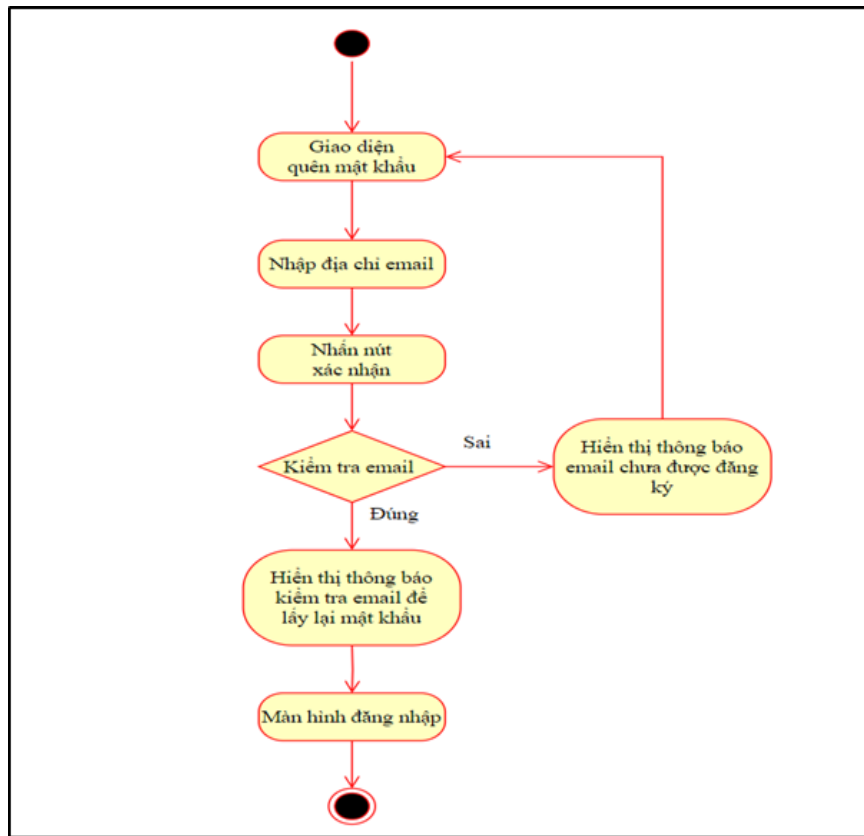
Hình 53. Sơ đồ bản vẽ hoạt động quên mật khẩu
