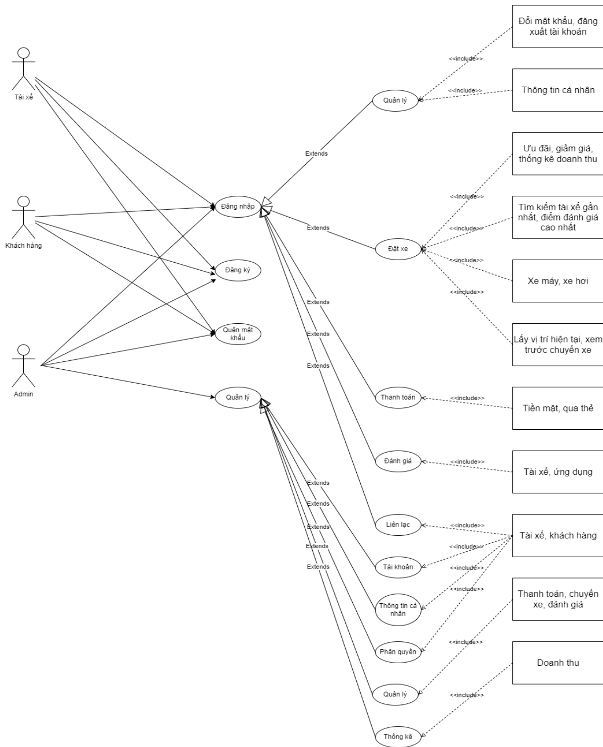
Hình 11. Sơ đồ Use Case tổng quát
