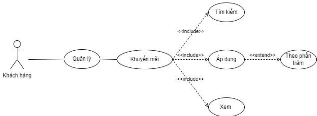
Hình 28. UseCase quản lý khuyến mãi
