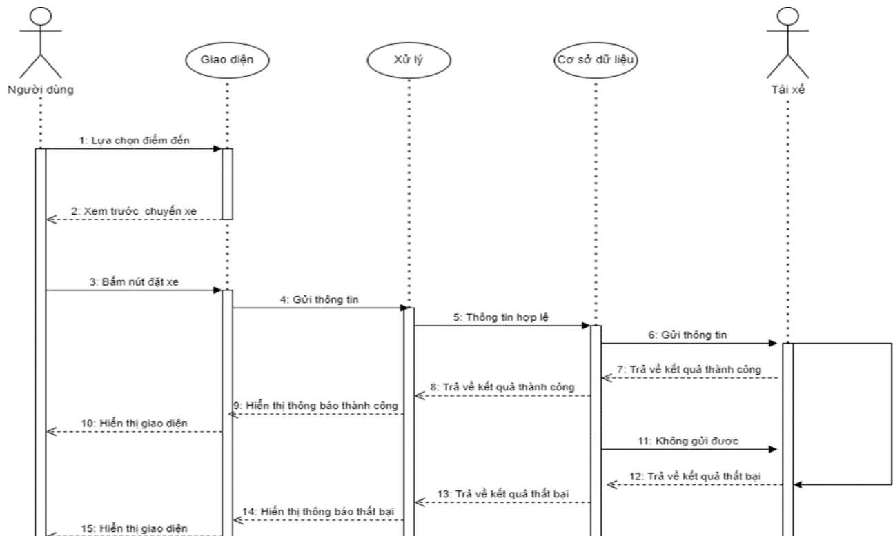
Hình 40. Sơ đồ tuần tự đặt xe
