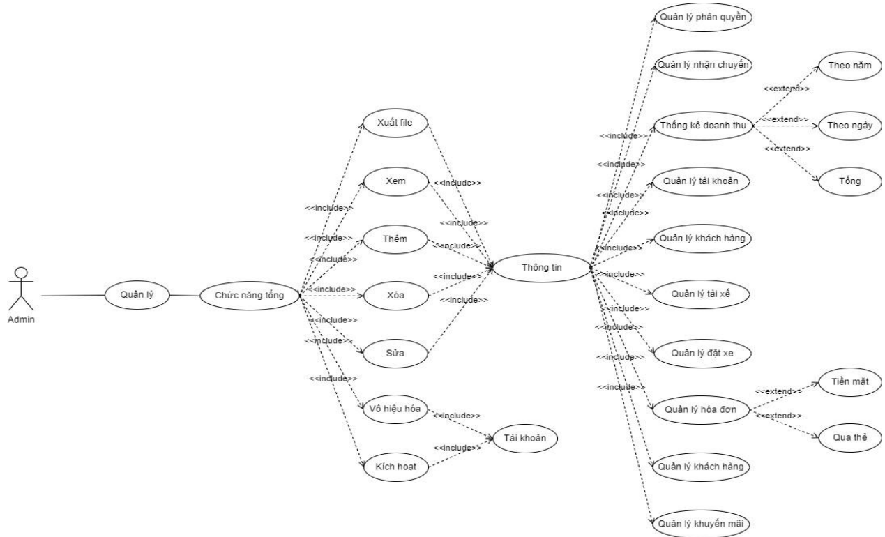
Hình 36. Đặc tả UseCase quản lý chức năng tổng
