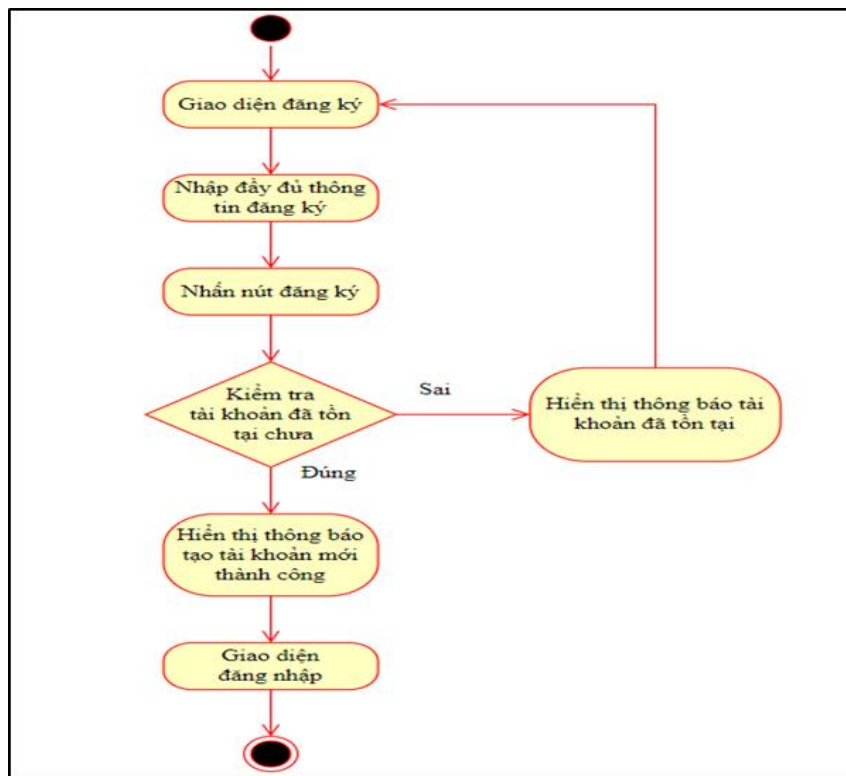
Hình 49. Sơ đồ bản vẽ hoạt động đăng ký
