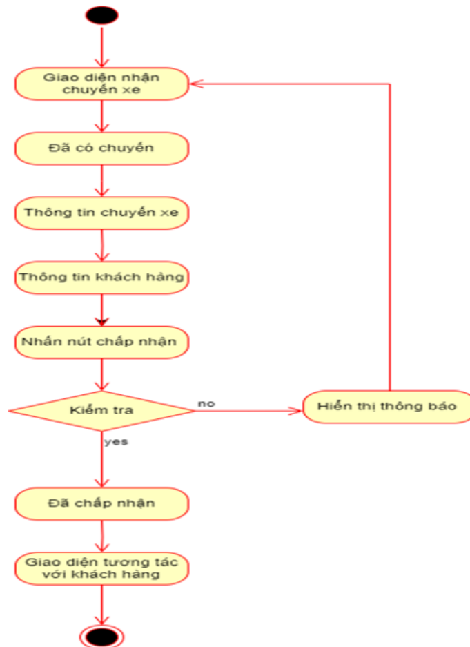
Hình 51. Sơ đồ bản vẽ hoạt động tài xế nhận chuyển xe
