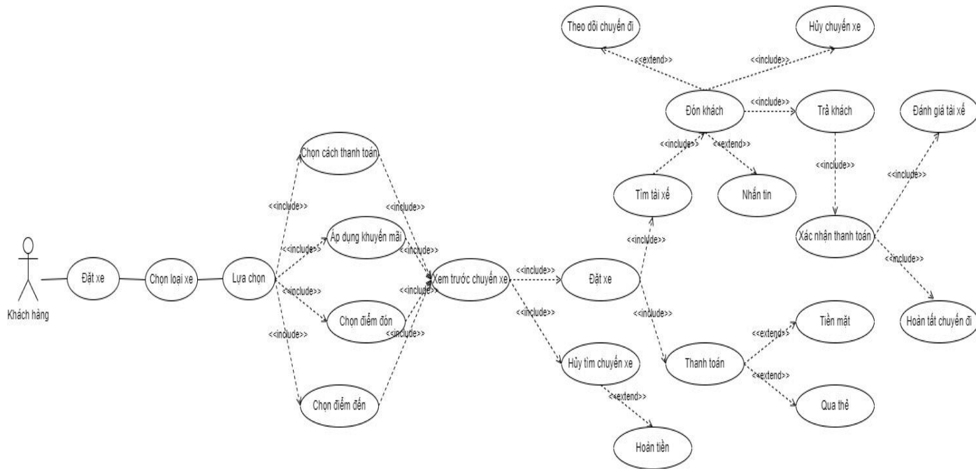
Hình 22. UseCase đặt xe
