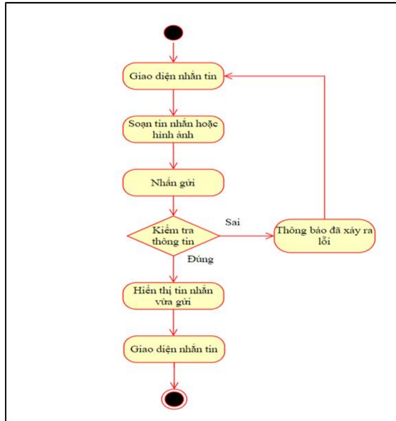
. Hình 52. Sơ đồ bản vẽ hoạt động nhắn tin
