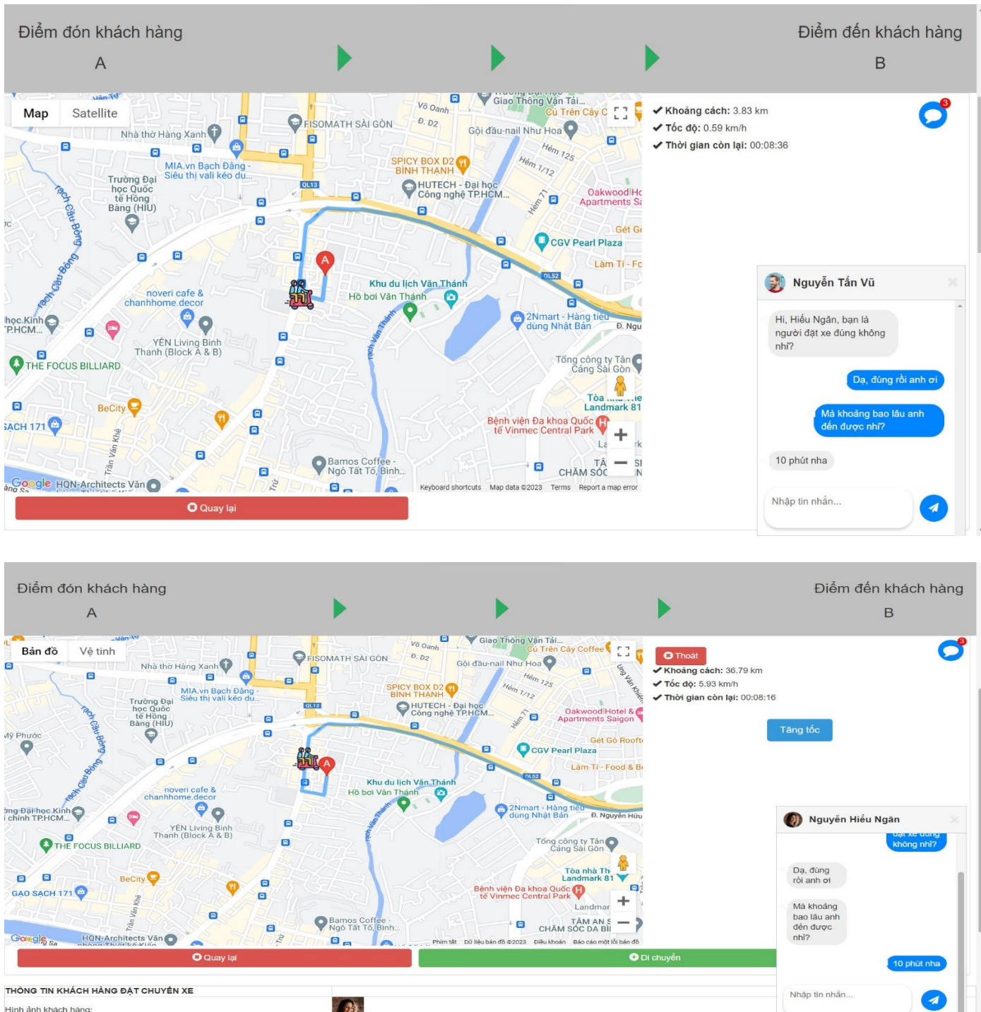
Hình 96. Màn hình theo dõi tài xế di chuyển tới điểm đến
