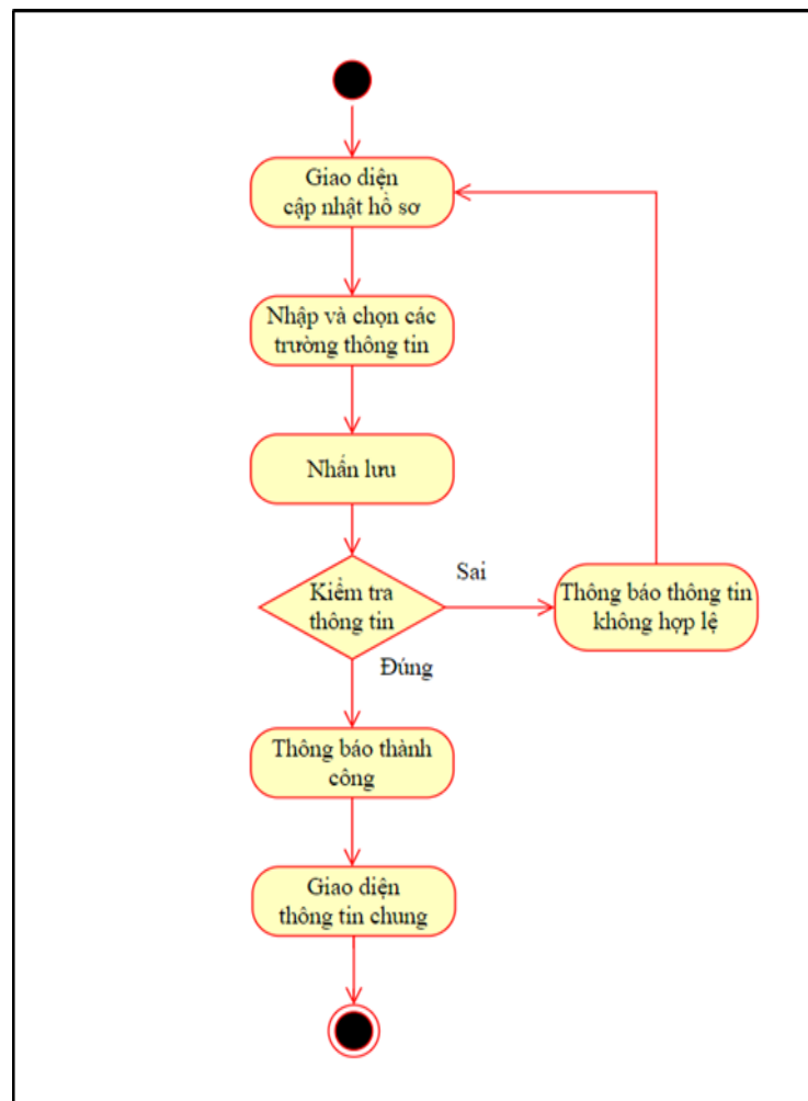
Hình 55. Sơ đồ bản vẽ hoạt động cập nhật thông tin cá nhân
